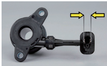
画像 1：LuK CSC 510 0090 10 油圧コネクタ 12.2 mm
