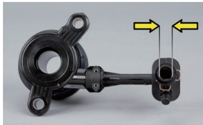
画像 3：LuK CSC 510 0098 10 油圧コネクタ 11.7 mm
