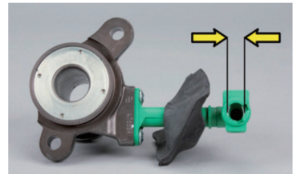
画像 2：LuK CSC 510 0097 10 油圧コネクタ 13.3 mm
